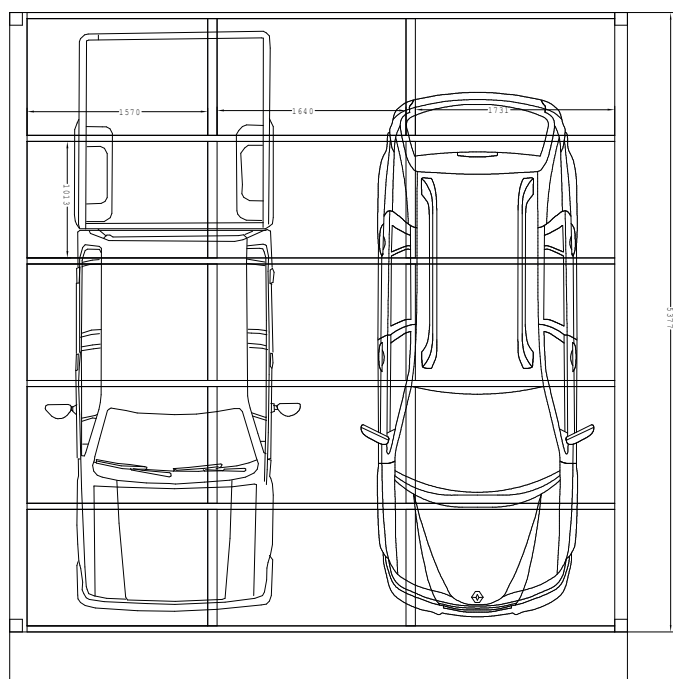
SAMONOSNÝ PRÍSTŘEŠEK 5377 x 5363 - SOLSOL PANELY
