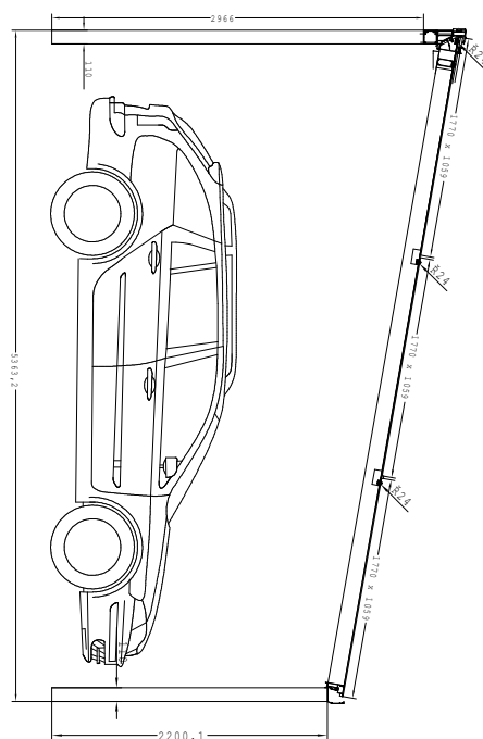
SAMONOSNÝ PŘÍSTŘEŠEK 5377 x 5363 - SOLSOL PANELY
