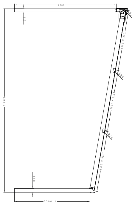
SAMONOSNÝ PRÍSTŘEŠEK 5377 x 5363 - SOLSOL PANELY
