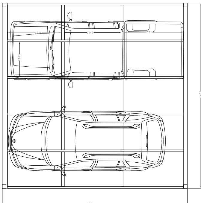
SAMONOSNÝ PŘÍSTŘEŠEK 5377 x 5363 - SOLSOL PANELY
